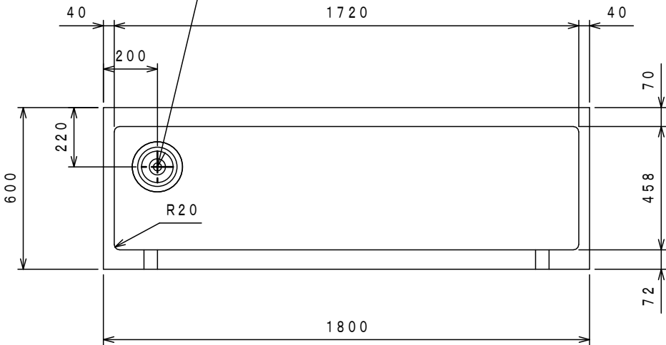
大型ゴミ収納器付防臭排水トラップ（４０Ａ）
