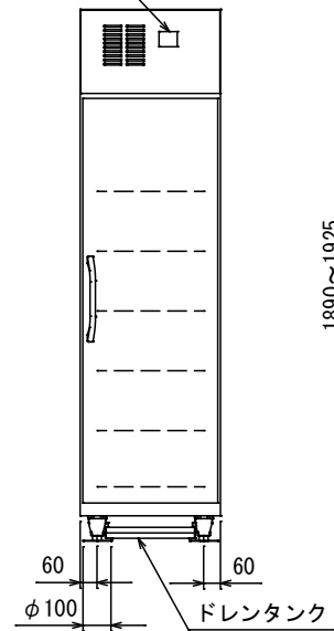
温度表示部
