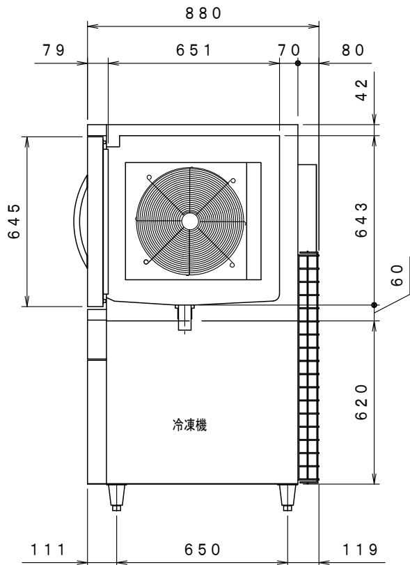
設置スペース図 (1 : 20)
